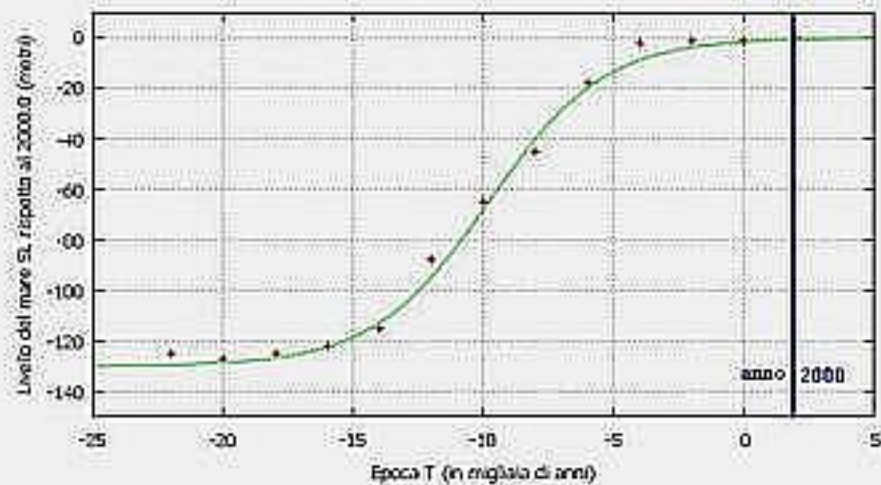
Variazione del livello marino negli ultimi 26000 anni
