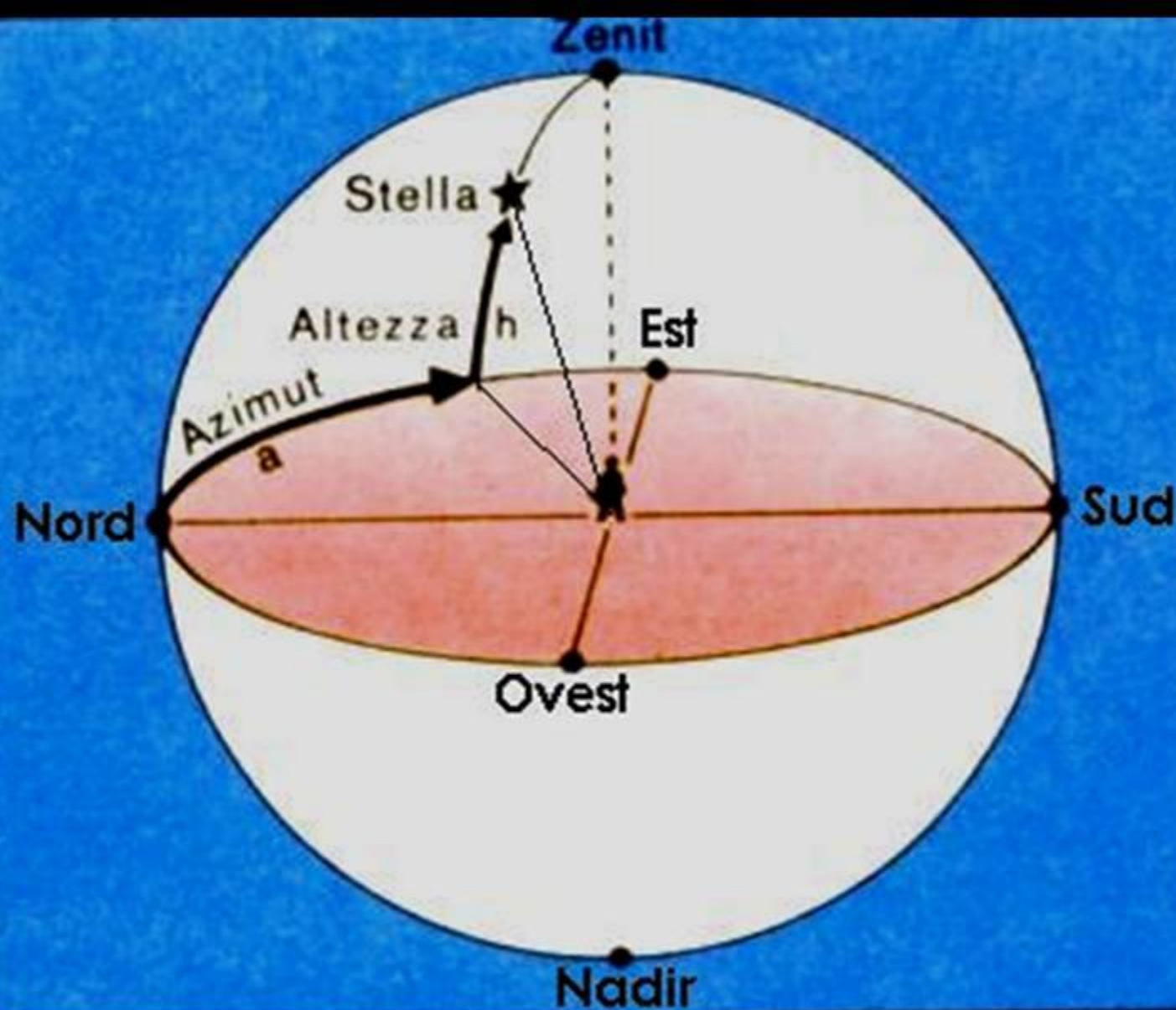
Sistema di Coordinate Altazimutale
